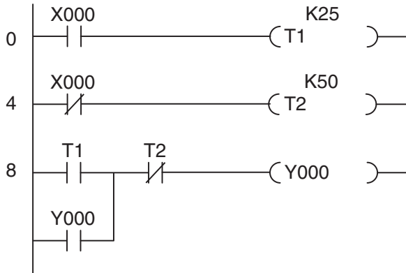
Létradiagram
