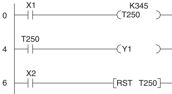
Létradiagram
