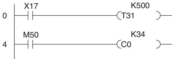
Létradiagram
