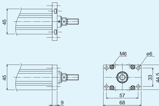
Abb. 16 Flanschplatte CT 45
