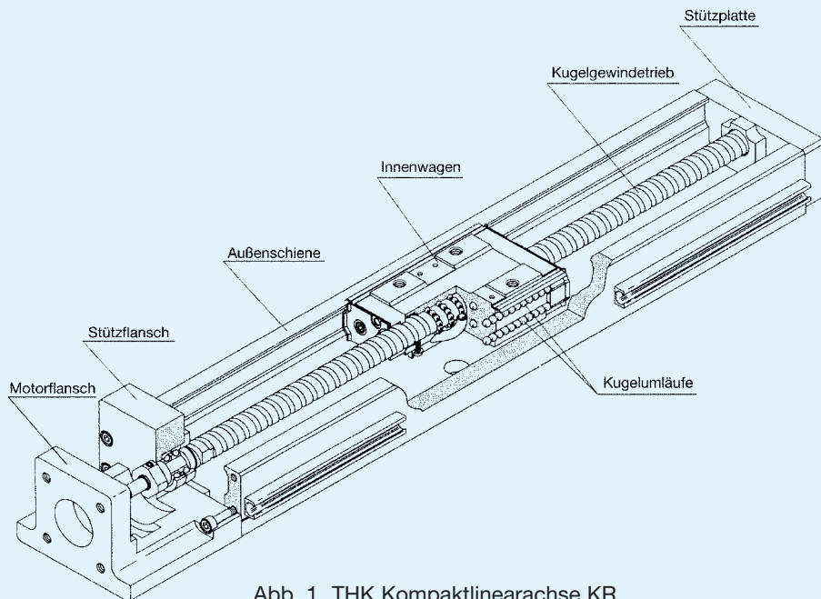
Abb. 1 THK Kompaktlinearachse KR
