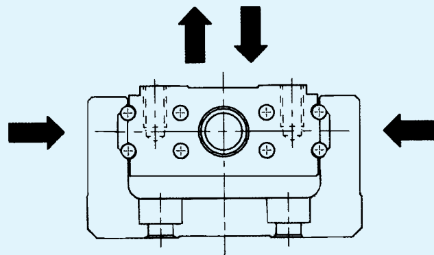
Abb. 2 Belastbarkeit KR
