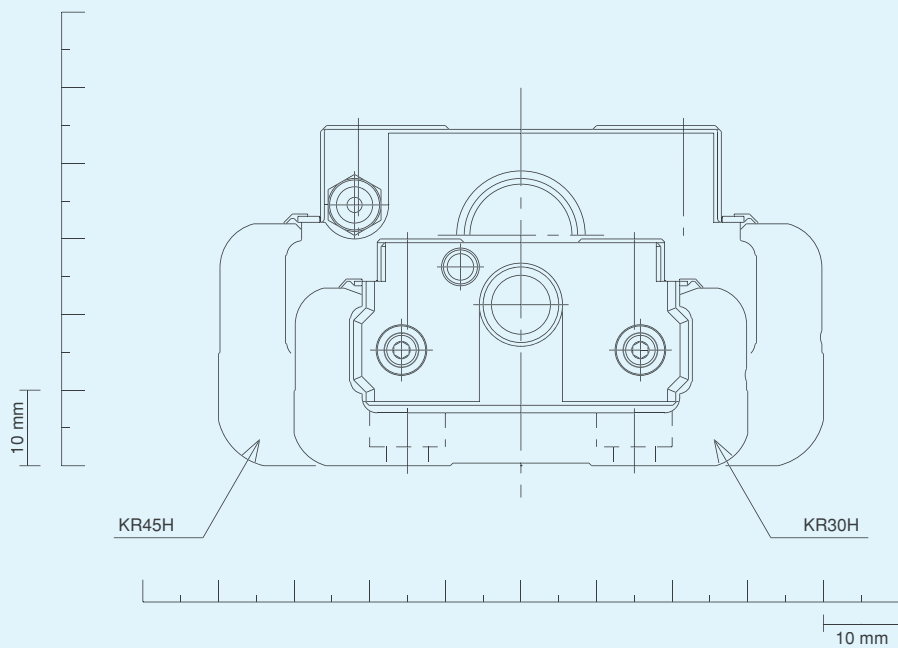
Abb.7 Querschnitt (Maßstab 1:1)
