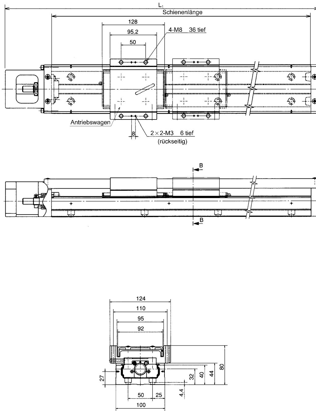
Querschnitt B-B
