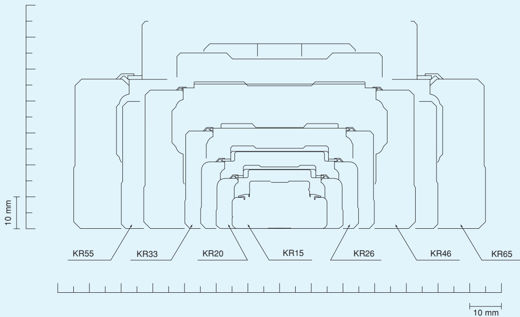
Abb.6 Die Baureihe KR im Querschnittsvergleich (Maßstab 1:1)
