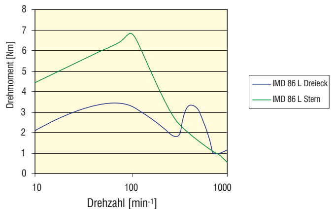
IMD 86 L
