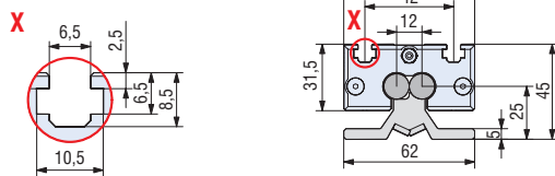
LFS-12-2 mit WS 4
