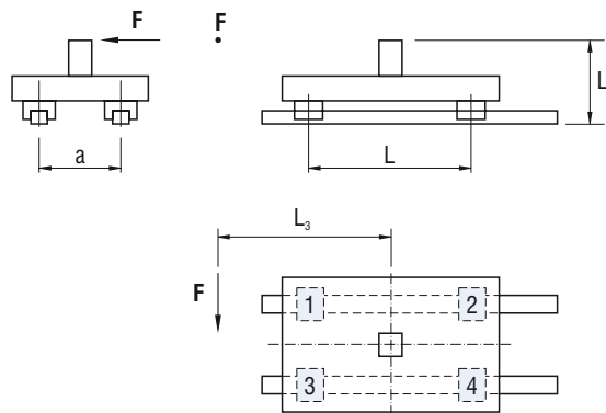
Maßbild
