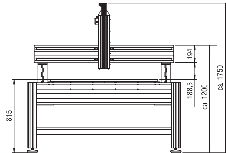
FLATCOM mit Untergestell, ohne Haube
