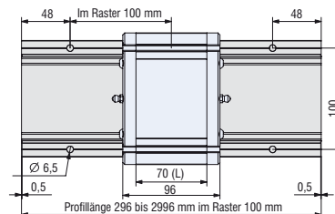
LFS-8-3 mit WS 3
