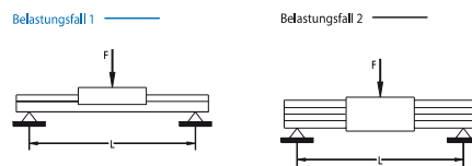
Durchbiegung Zahnriemenvorschub LEZ 2
