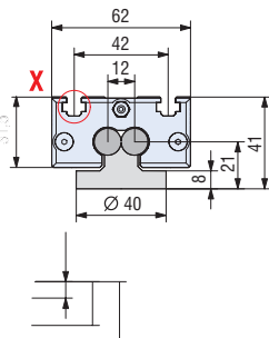
LFS-12-1 mit WS 4
