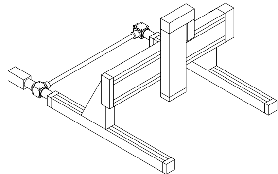
3-Achs-Flachbettanordnung 2 x LES 4, LES 5, LES 6, 2 x PS 2, 2 x WV 2 Winkelgetriebebesatz, PS 4, PS 7
