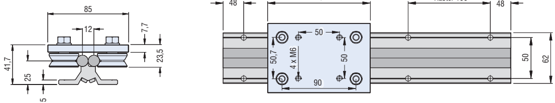
LFS-12-2 mit LW 3
