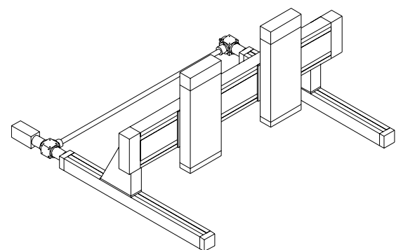
5-Achs-Flachbettanordnung 2 x LES 5 (Z-Achsen) LES 5 (2 Spindeltriebe) 2 x LES 4, 2 x PS 2, 2 x WV 2 Winkelgetriebebesatz, 2 x PS 4 mit VP 2
