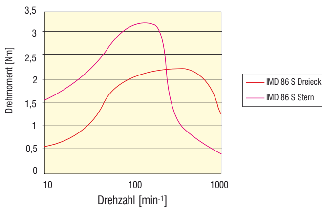
IMD 86 S
