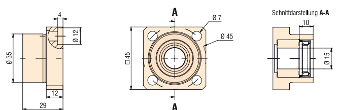
Flanschlager Loslagerseite
