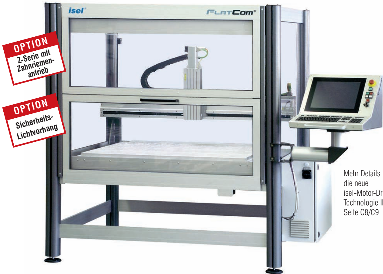
FLATCOM mit geschlossener Haube
