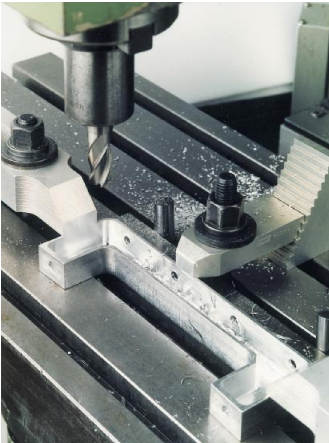
Alu-Spannpratzen im Einsatz
