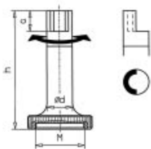
Aufsatzteil 180°, abgesetzt drehbar
