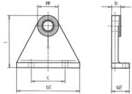
Zeichnung zeigt Fuß #82797 in Posifix-Systemgröße 50
