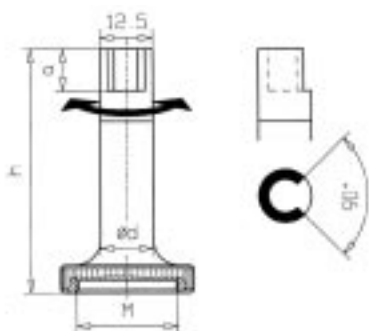
Aufsatzteil 90°, abgesetzt drehbar
