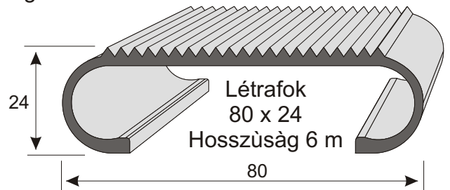
Létrafok 80 x 24 Hosszúság 6 m Körszelvényű cső 16 mm 16x4 vagy 16x3 mm méretű csövek becsipenthetők
