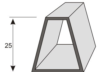
P9254 Trapéz cső 25x22x10x1,2 Hosszúság 6 m
