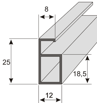
P17 szűnyogháló profil Hosszúság 6 m
