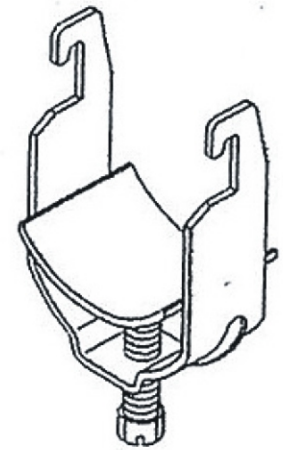
kengyel csöbilincs horganyzott acél
