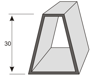
P9227 Trapéz cső 30x25x10x1,3 Hosszúság 6 m
