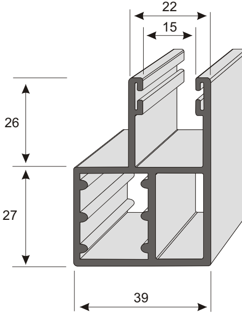
B07 speciális profil 53 x 39 Hosszúság 6 m
