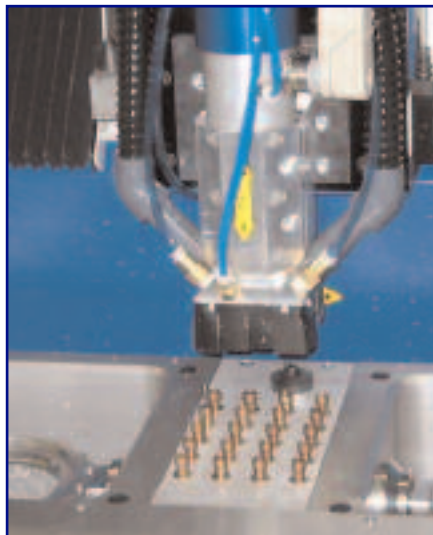
HF-Spindel mit Sonder-Werkzeugwechsler / HF motor speciális szerszámcsere
