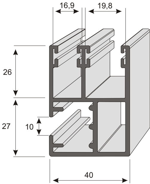
B09 speciális profil 53 x 40 Hosszúság 6 m
