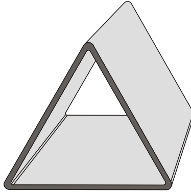
D70 Háromszögletű zártszelvény 70 x 70 x 1,2 Hosszúság 6 m
