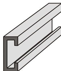
P245 C-Profil 24,5 x 10 x 2 nyílás 14,5 mm Hosszúság 6 m
