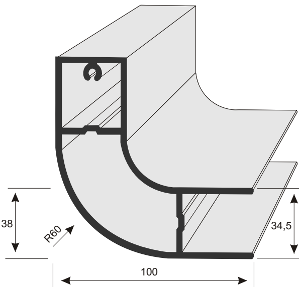
P9160 aláfutásgátló szegő - profil 100x100x34,5x1,8 mm Hosszúság 6 m
