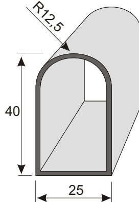
P9231 díszítő keretprofil 40 x 25 x 1,3 Hosszúság 6 m
