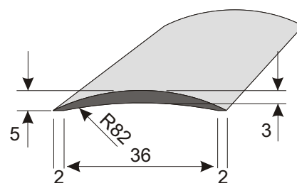
áthidaló speciális profil 40 x 5 mm Hosszúság = 6,5 m
