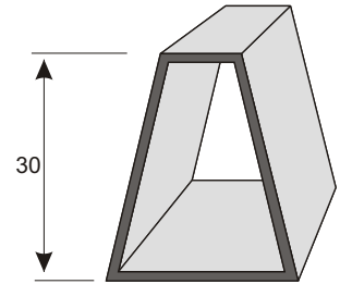
P9227 Trapéz cső 30x25x10x1,3 Hosszúság 6 m
