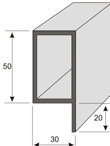
P70 zártszelvény 70 x 50 x 30 x 2 Hosszúság 6 m
