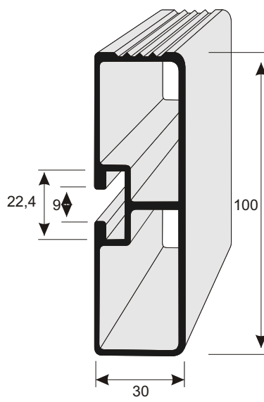
P9161 oldal aláfutásgátló - profil 100x30x2 mm, eloxált A6C0 Hosszúság 7,2 m
