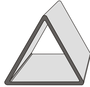
D50 Háromszögletű zártszelvény 50 x 50 x 1,5 Hosszúság 6 m
