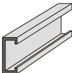
P03 C-Profil 25 x 10 x 1,5 nyílás 18 mm Hosszúság 6 m
