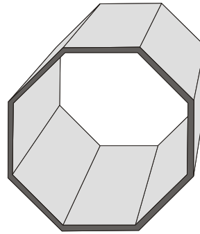
A60 Nyolcszög profil 60 x 1,5 Hosszúság 6 m
