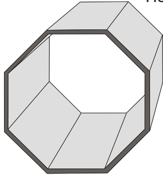
A72 Nyolcszög profil 72 x 2,5 Hosszúság 6 m
