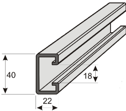
ankersin 40 x 22 A8 gelocht Nyílás 18 mm horganyzott acél Hosszúság 6 m és 2 m
