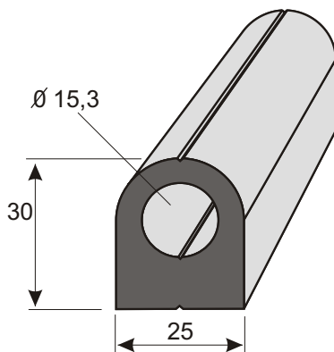
P05 30 x 25 Hosszúság 6 m
