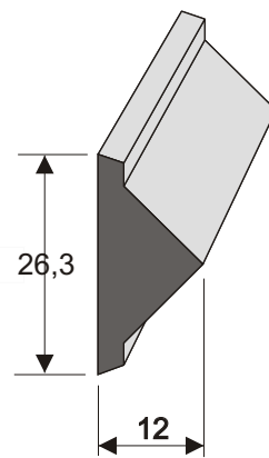
P07 szegély Hosszúság 7,75 m
