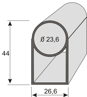
P23 44 x 26,6 x 1,2 Hosszúság 6 m
