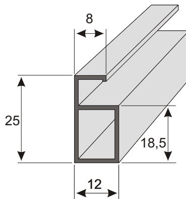
P17 szűnyogháló profil Hosszúság 6 m
