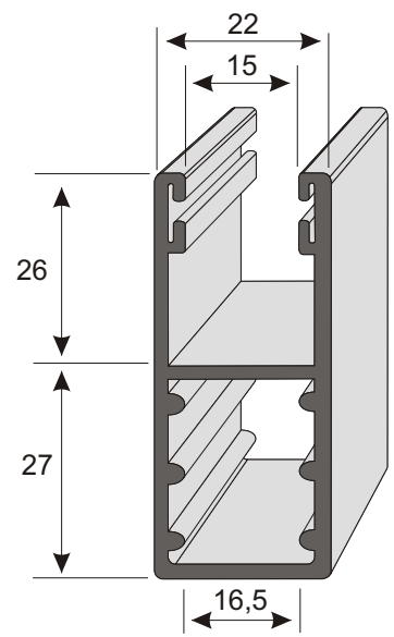
B01 speciális profil 53 x 22 Hosszúság 6 m
