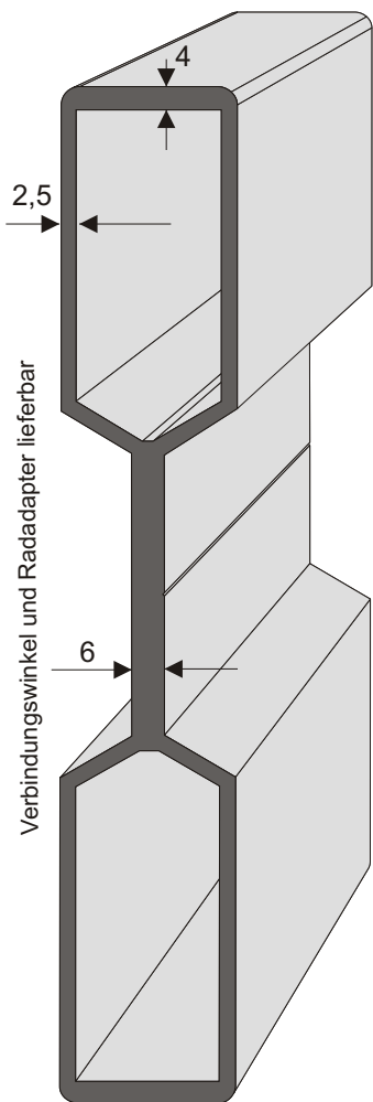
P Z175 Tok 175x30
