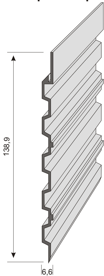
P 9256 fedőprofil 139 x 6,6 Hosszúság 6 m
