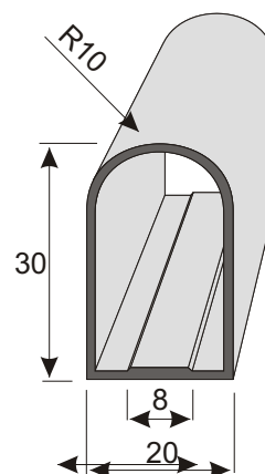
P9268 díszítő keretprofil 30 x 20 x 1,3 Hosszúság 6 m
