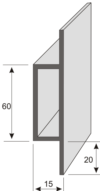
P60 zártszelvény 100 x 60 x 15 x 2 Hosszúság 6 m
