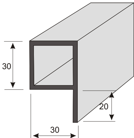
P51 zártszelvény 50 x 30 x 30 x 2 Hosszúság 6 m
