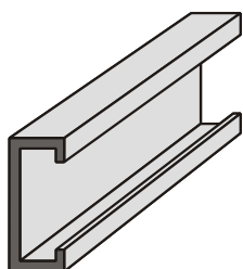
P24 C-Profil 24,3 x 10 x 1,5 nyílás 19,1 mm Hosszúság 6 m
