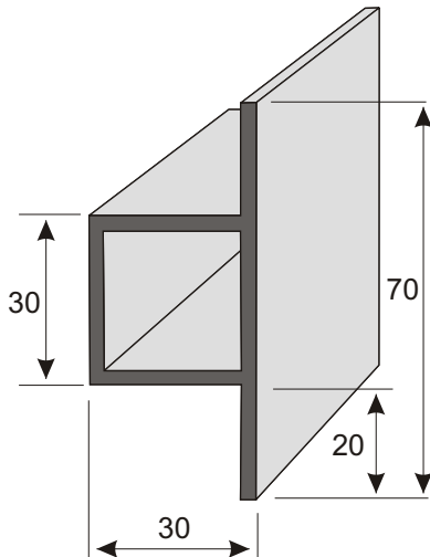
P73 zártszelvény 70 x 30 x 30 x 2 Hosszúság 6 m
