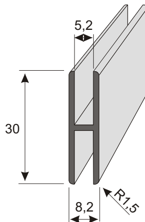
P20160 H-profilok Hosszúság 6 m
