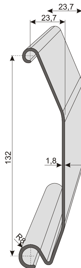
P-R 132 tolókapuprofil Hosszúság 6120 mm
