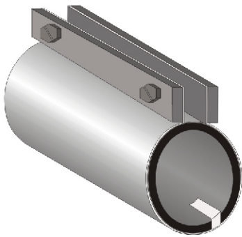
csöbilincs két csavarral M8 1.4016 / Gumi EPDM földelőszalaggal Hosszúság = 100 mm
