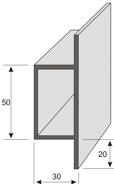
P93 zártszelvény 90 x 50 x 30 x 2 Hosszúság 6 m
