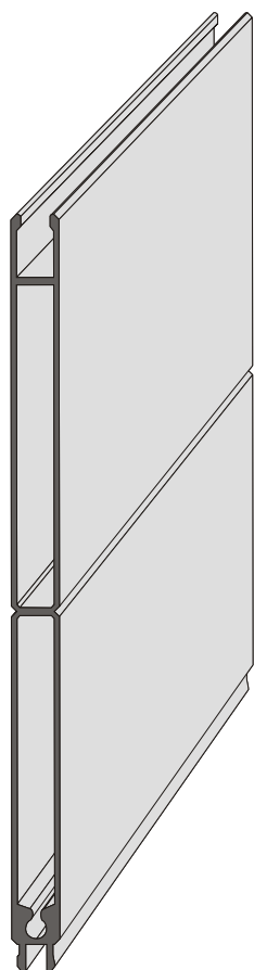
P 9279 átlátás elleni védelem 124 x 8,5 Hosszúság 6 m
