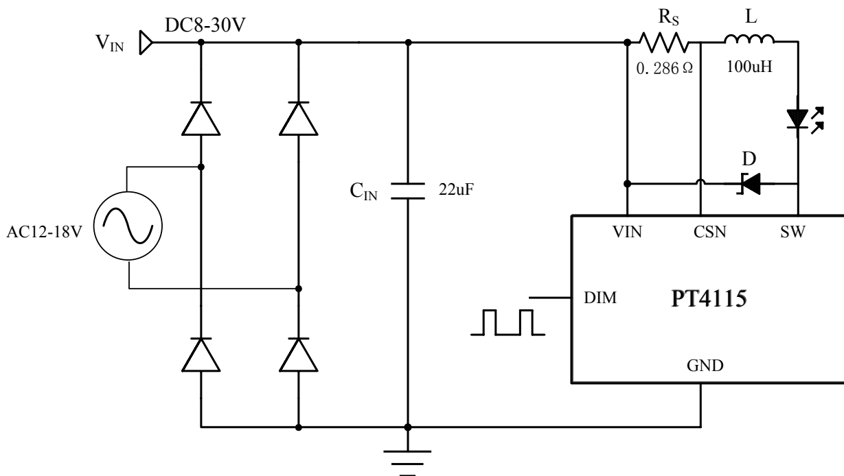
Fig1 : 1W application
