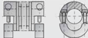
Miniaturkupplung in Halbschalenbauweise
