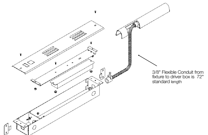
Type H Wiring Option: flexible conduit
