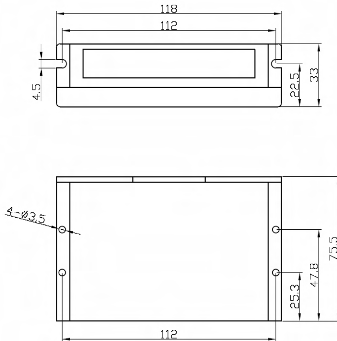
1. ábra: Mechanikai méretek
