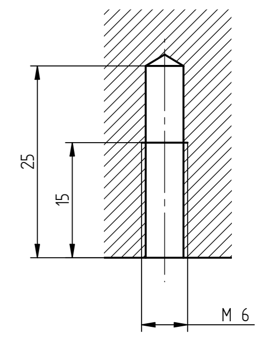
B-B M 2 : 1
