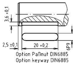
Paßfeder / key A6x6x20 DIN6885
