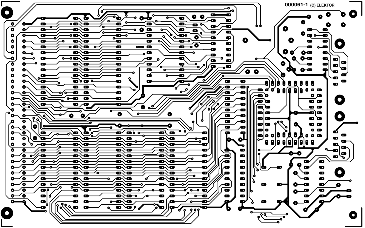
soldeerzijde
