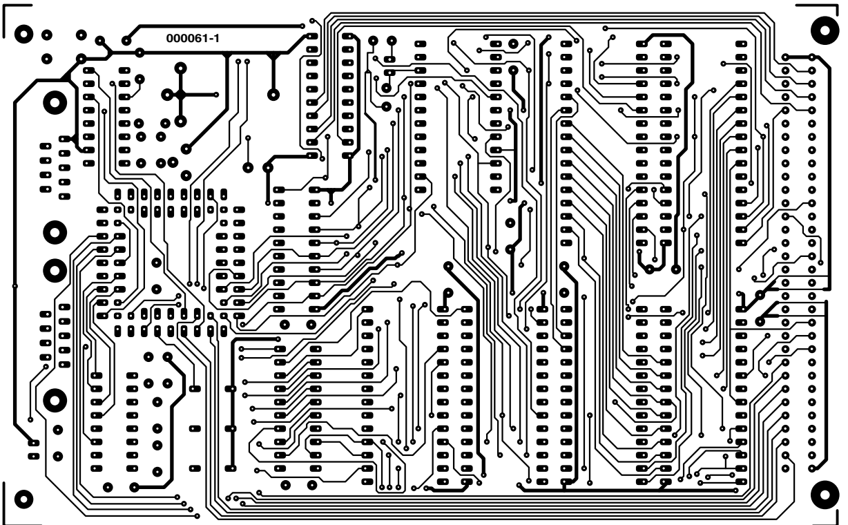
componentenzijde
