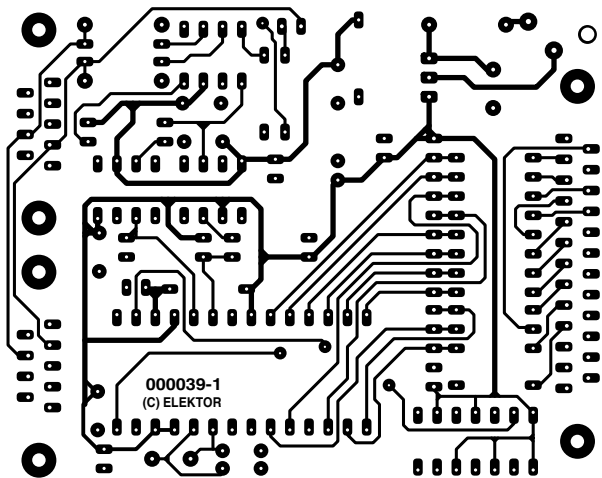
soldeerzijde
