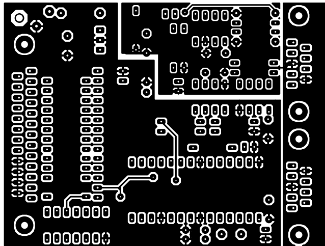
componentenzijde
