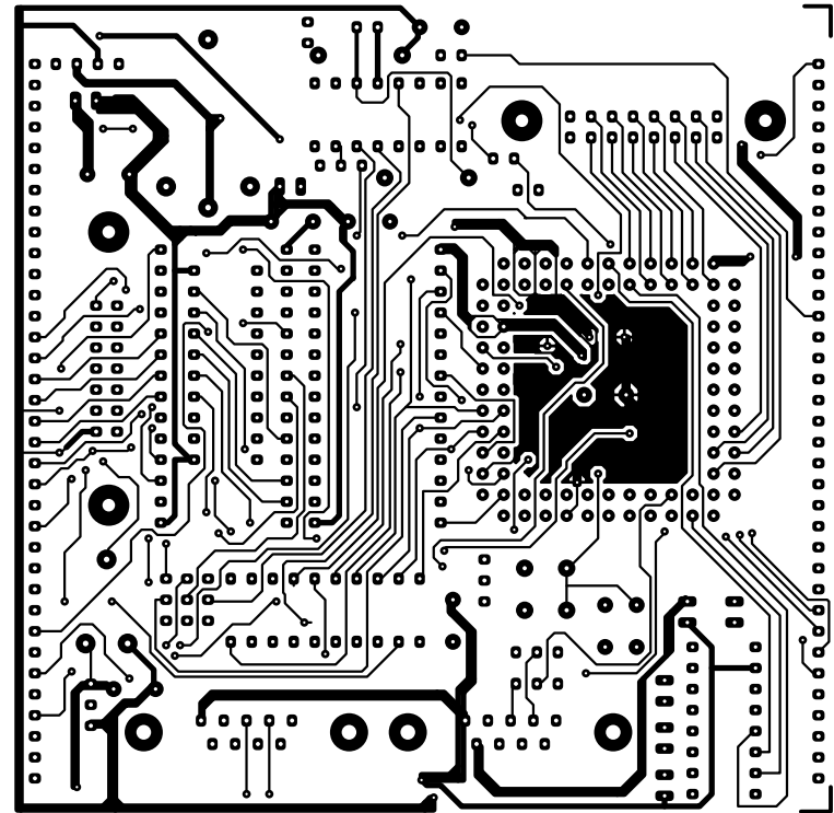
componentenzijde
