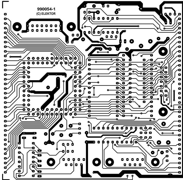
soldeerzijde
