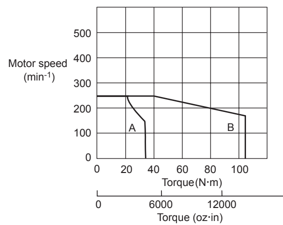
SGMCS-35E
