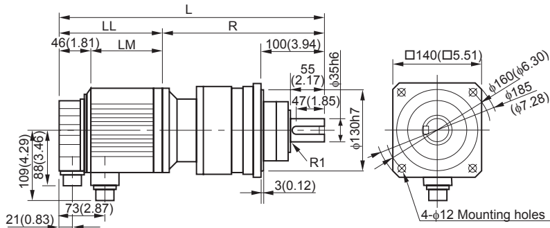
ANFJ-L30
