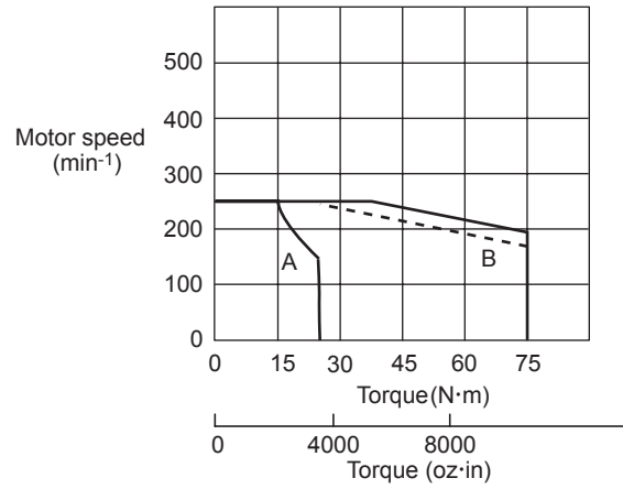
SGMCS-35E
