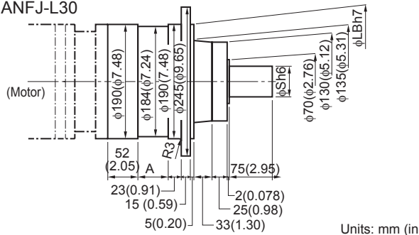
ANFJ-L30
