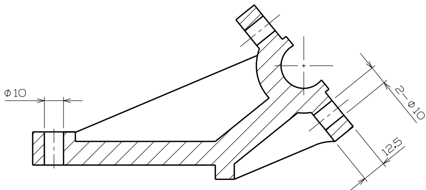
단면 A-A
