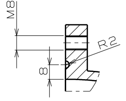
섹션 뷰 B-B
