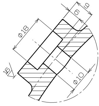
세부사양 축척 (2 : 1)
