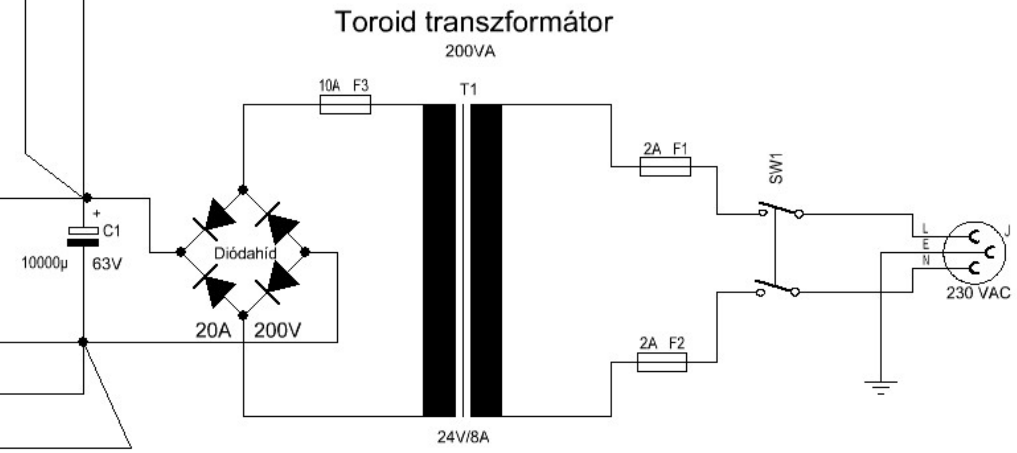
3 tengelyes vezérlő kapcsolási rajza
